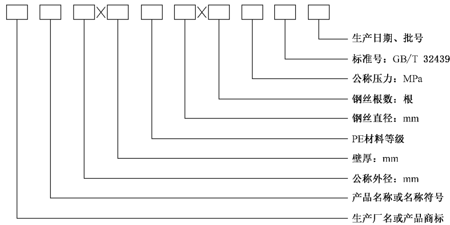
图 4 管材标志图
