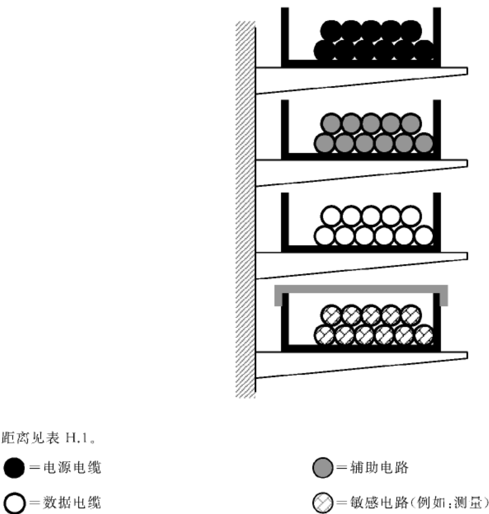
图 H.2 垂直分离和隔离的例子
