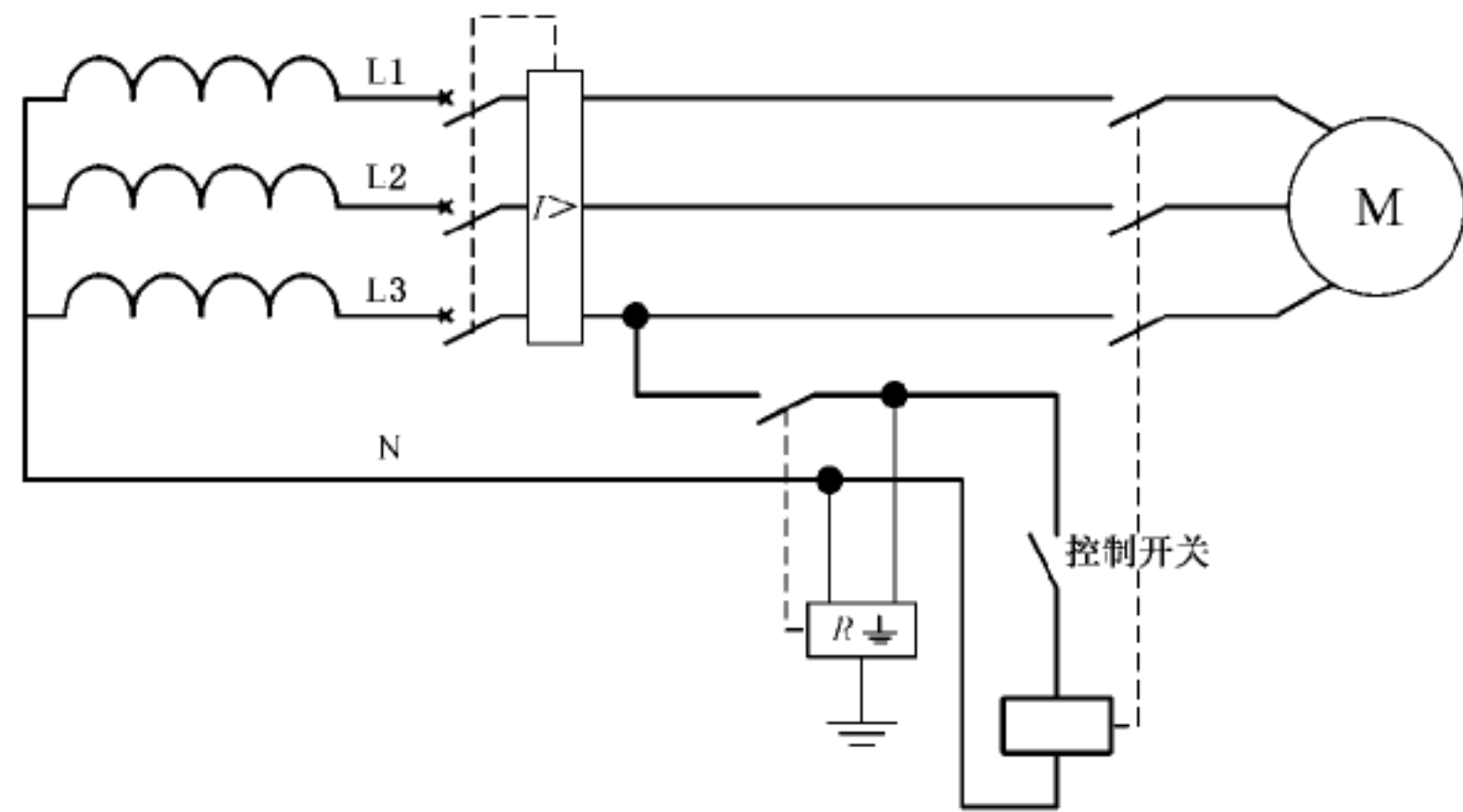
图 14 方法 d)2)a)不接地系统相线和中线之间控制电路没有连接变压器
