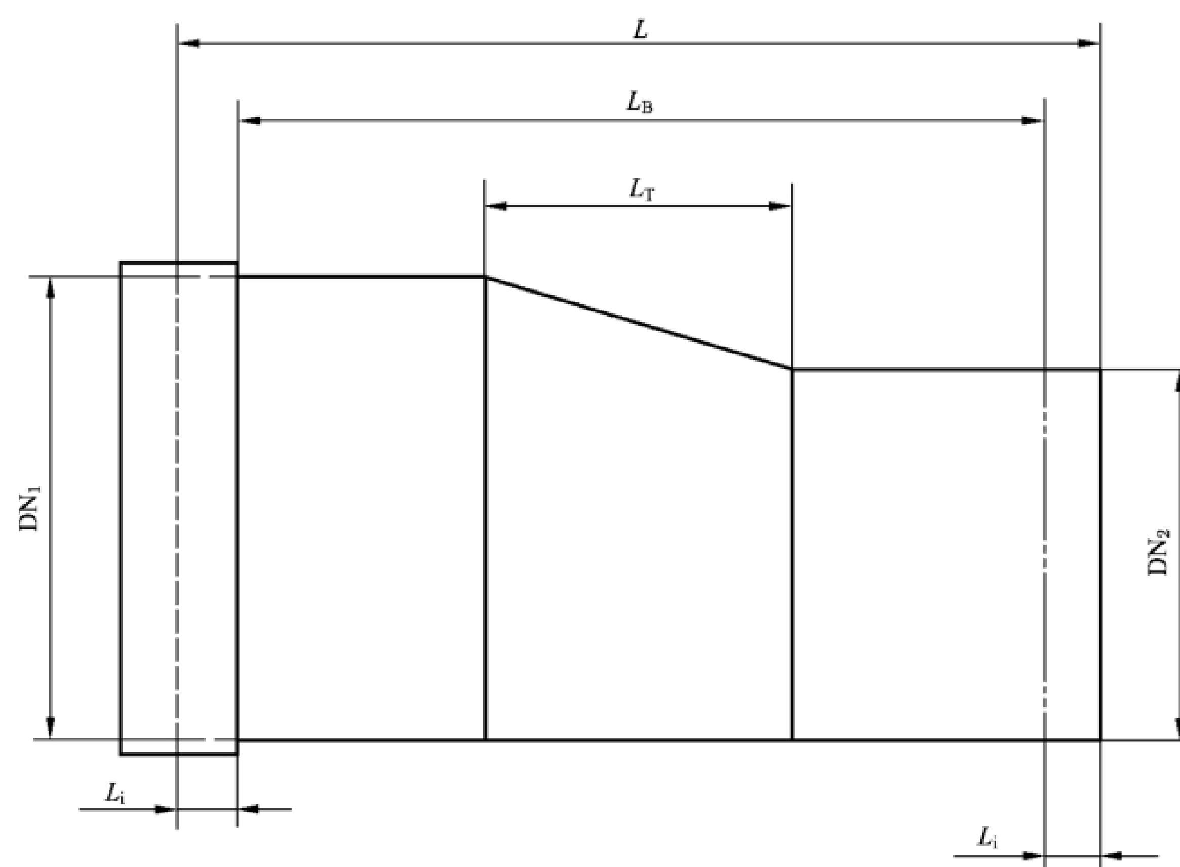
b) 偏心变径管
