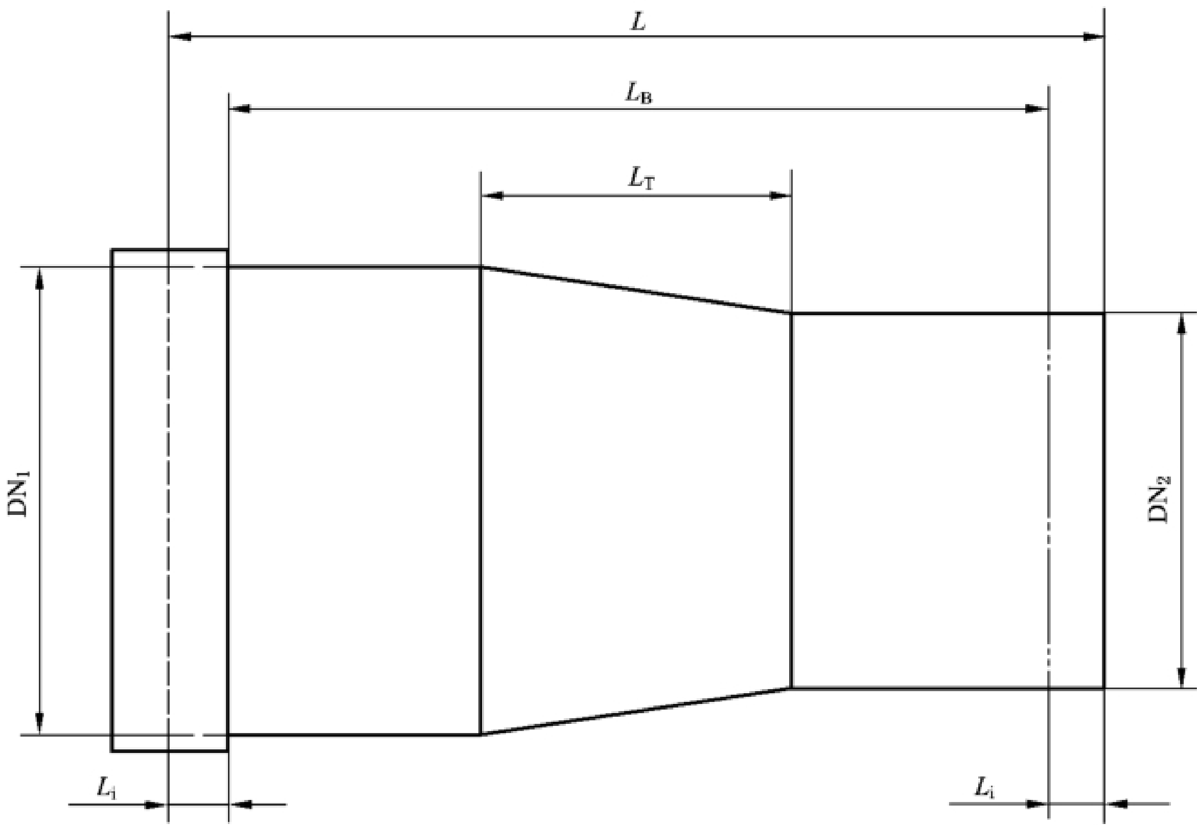
a) 同心变径管
