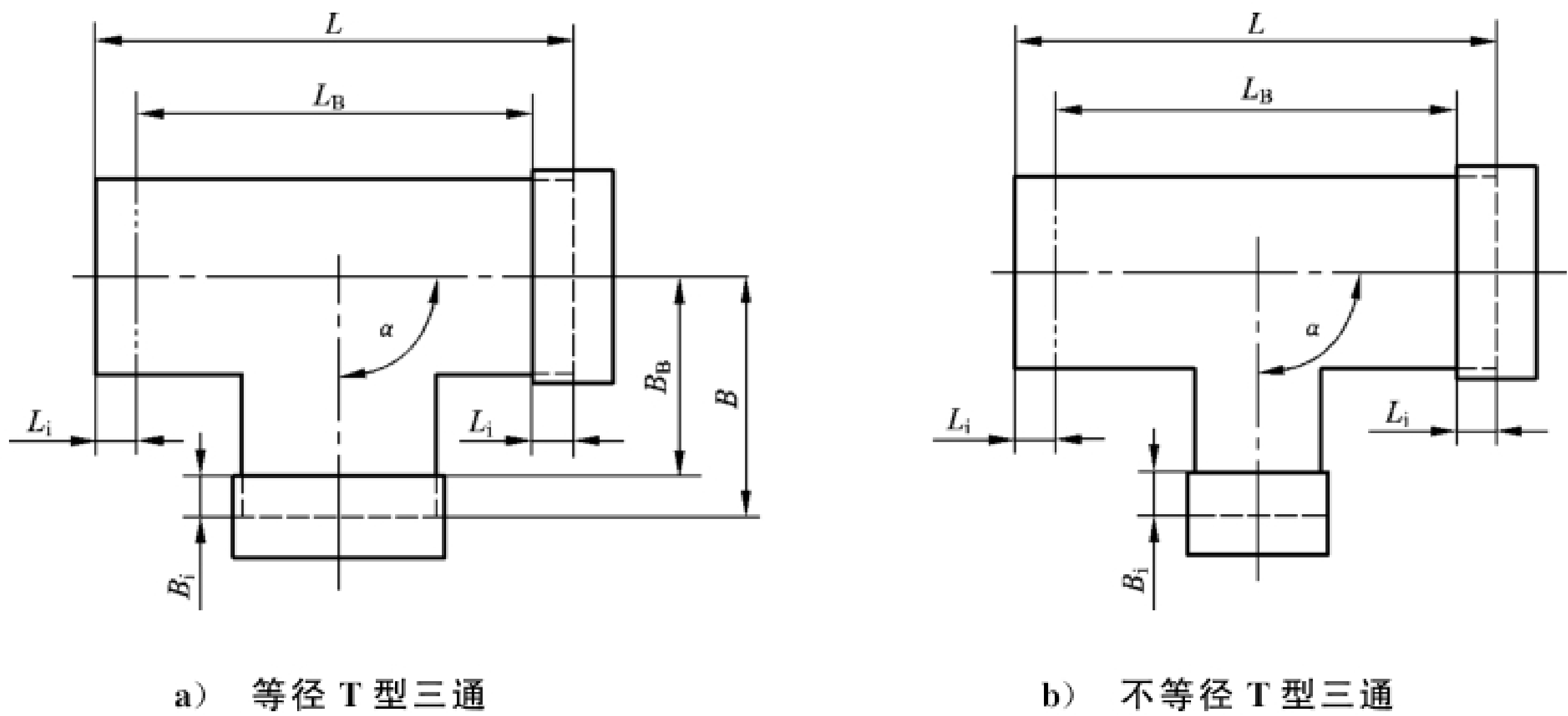
图 E.3 典型的三通
