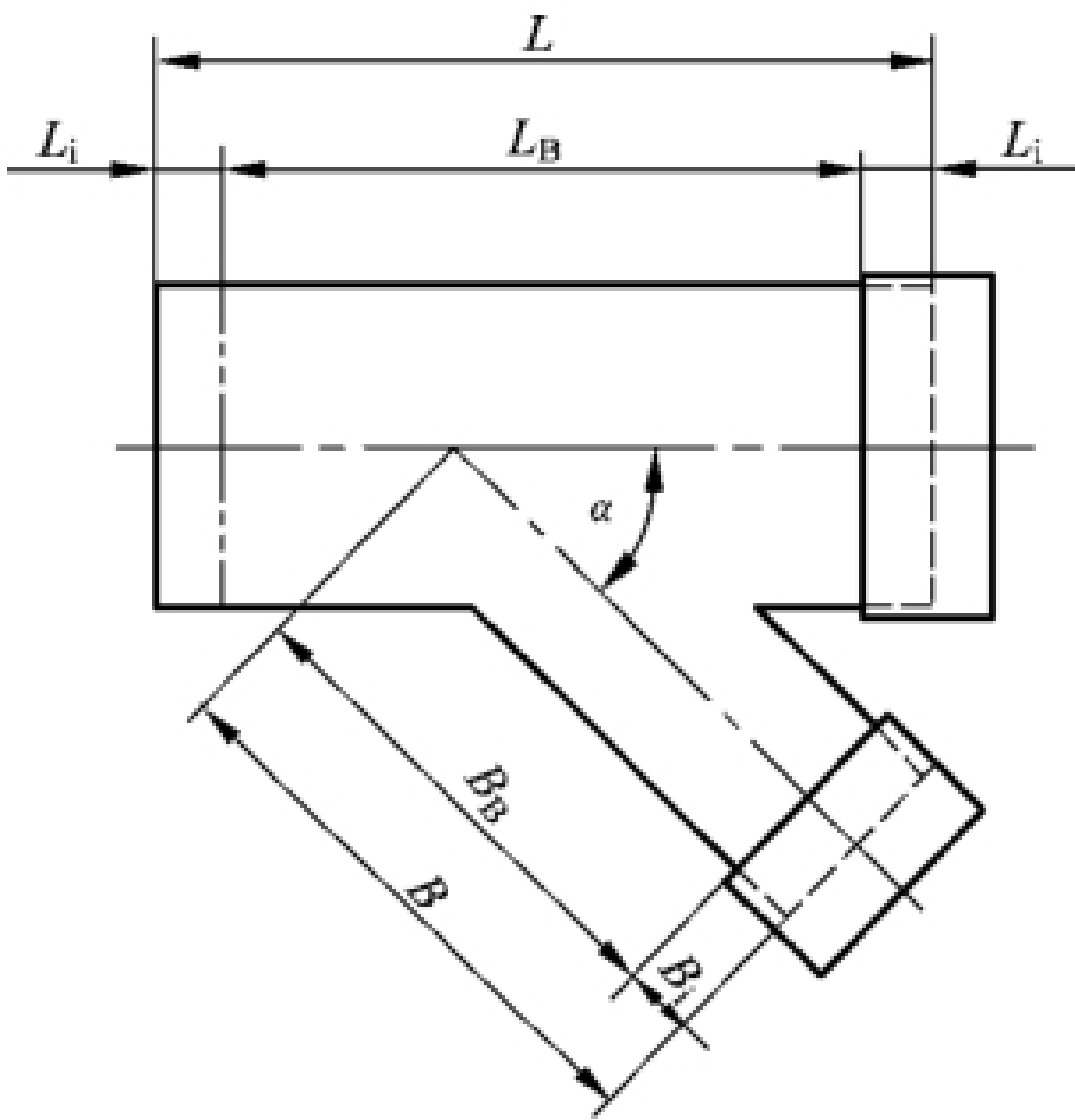
c) 不等径斜三通
