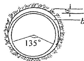
图 6.3.7 超挖示意图
