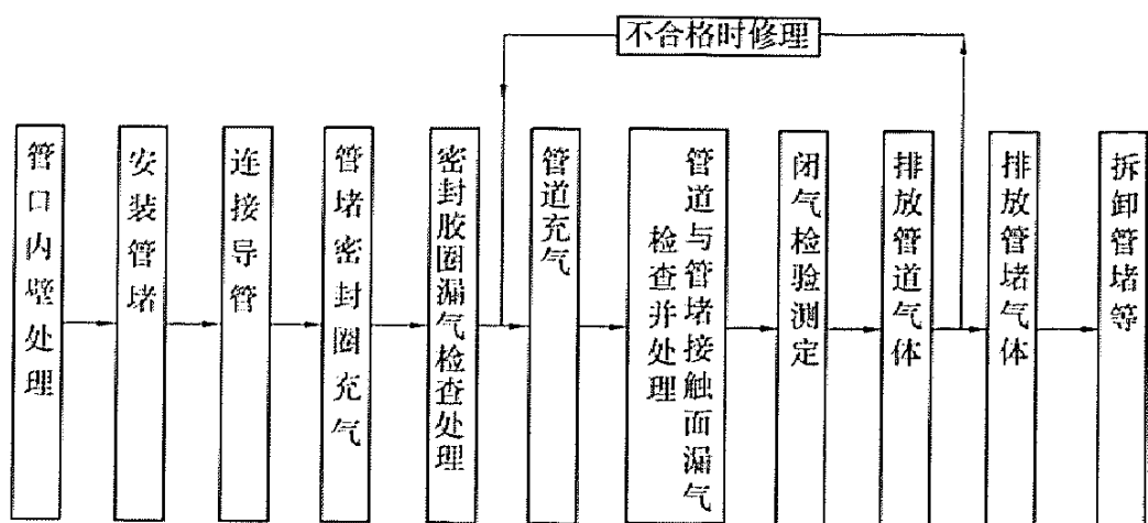
图 E. 0. 2 管道闭气检验工艺流程图
