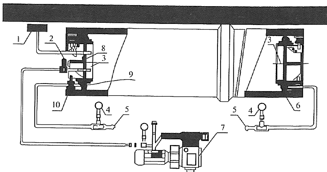
图 E. 0.1 排水管道闭气检验装置图
