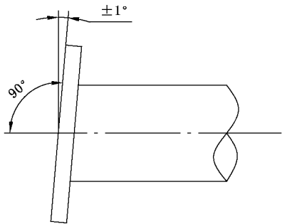
图 1 法兰平面与钢管轴线垂直度示意图
