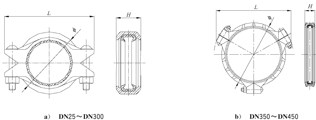
图 C.3 柔性管接头
